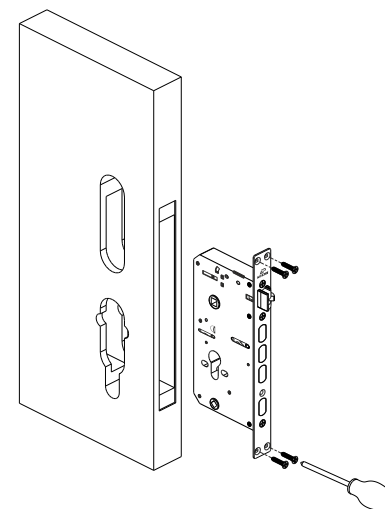
Рисунок №4. – Установка врезного механизма замка
