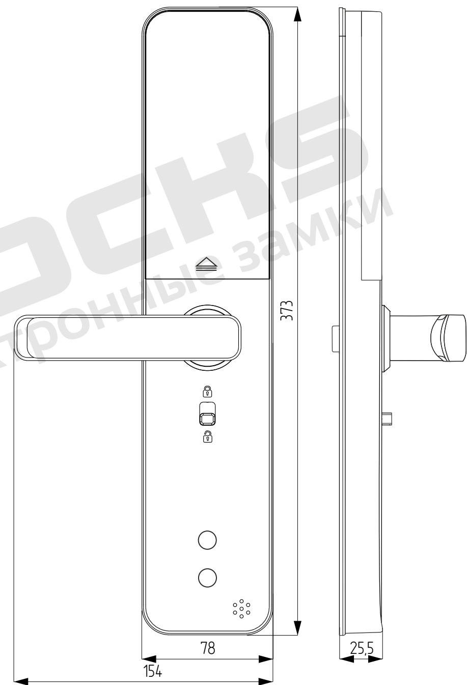
Внутренняя панель
