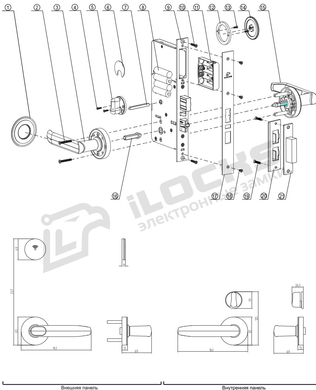
Рисунок №1 – Структурная схема (спецификация) замков типа iLOCKS IS190
