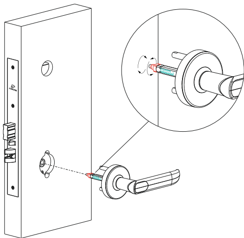
Рисунок №4 – Регулировка квадрата и установка передней (внешней) ручки
