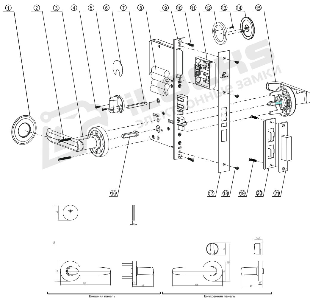
Рисунок №1 – Структурная схема(спецификация) замков типа iLOCKS IS190
