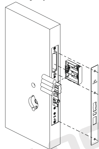
Рисунок №3 – Установка батареек типа АА
