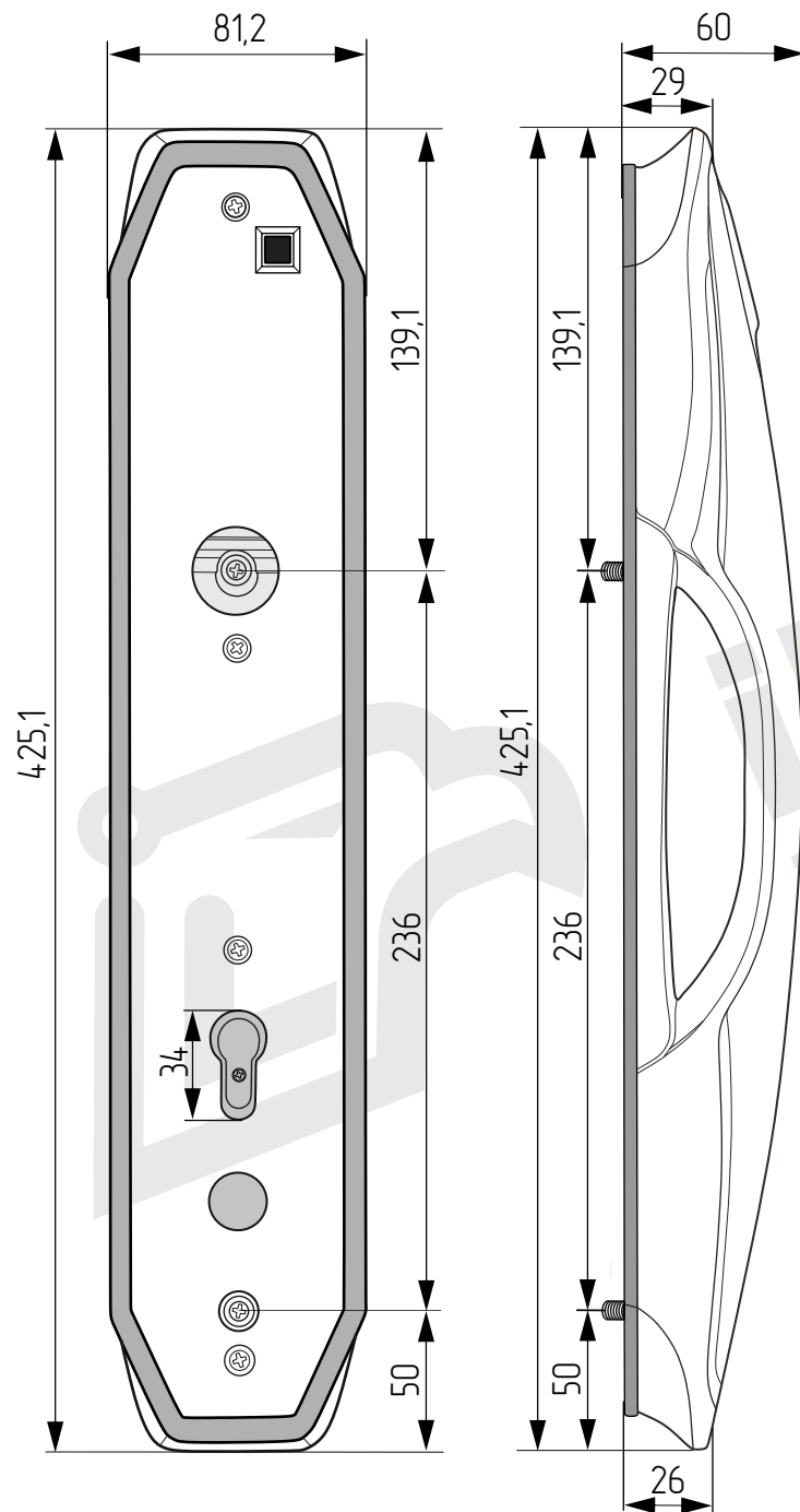
Внешняя панель
