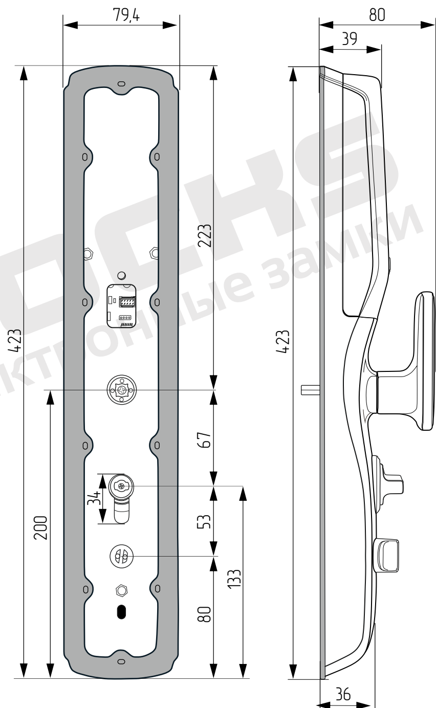
Внутренняя панель
